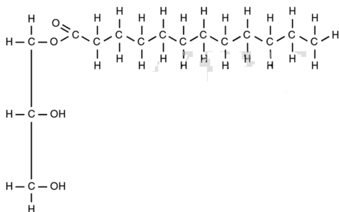
(b) Monoglyceride
